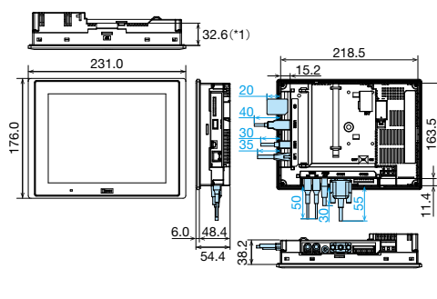
HG3G-V8形 (8.4インチ)
