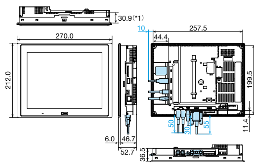
HG3G-VA形 (10.4インチ)
