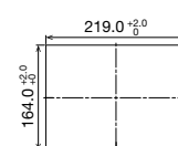
HG3G-V8形 (8.4インチ)
