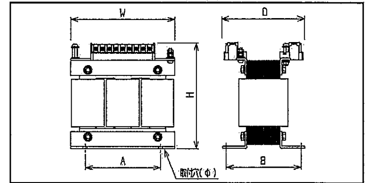
寸法確認図
