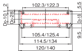
A-A(AGS-12□□10-SQまたはAGS-14□□10-SQの場合)
