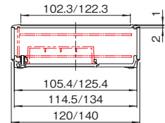
B-B(AGS-12□□10-SQまたはAGS-14□□10-SQの場合)
