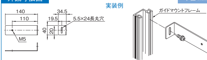
標準取付位置 ラック内部(ガイドフレーム/Hフレーム)
