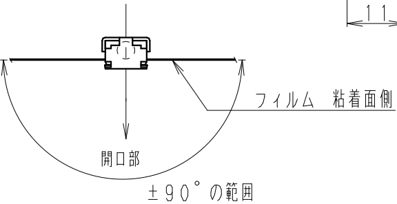
矢視 A (3:1) U.FL(A) コネクタ向き
