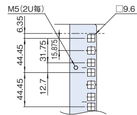
A部詳細
