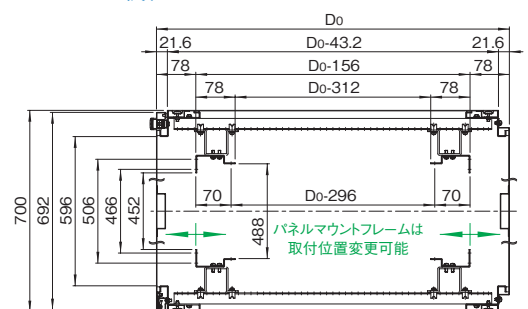
B-B
