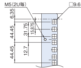
A部詳細
