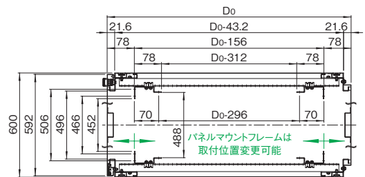
B-B
