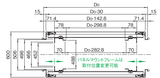
B-B
