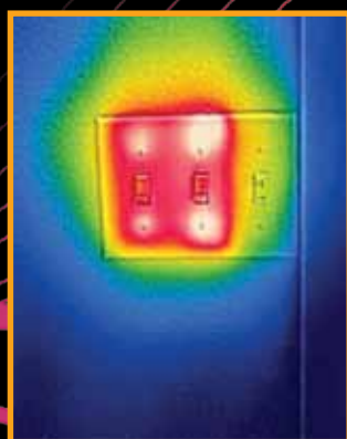
電気器具のホットスポット
