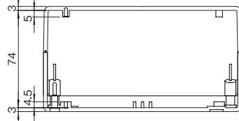
鉛直断面(側面)
