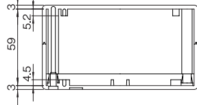
鉛直断面(側面)
