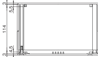
鉛直断面(側面)
