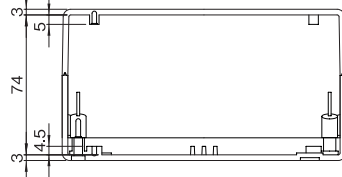
鉛直断面(側面)
