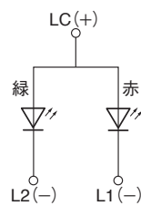
超高輝度LED(輝度レベル2) 周囲温度 Ta=25°C
