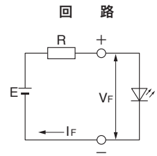
LED回路の制限抵抗について
