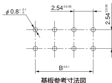
基板参考寸法図
