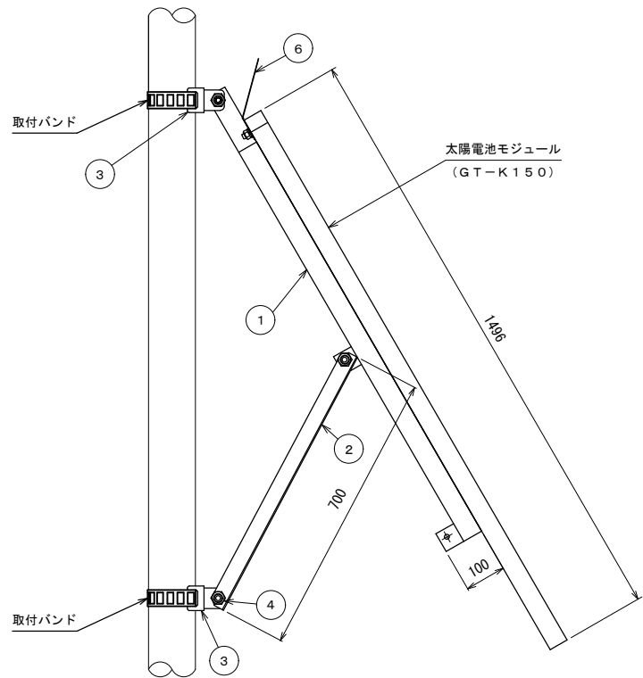
架台全体図 太陽電池60°
