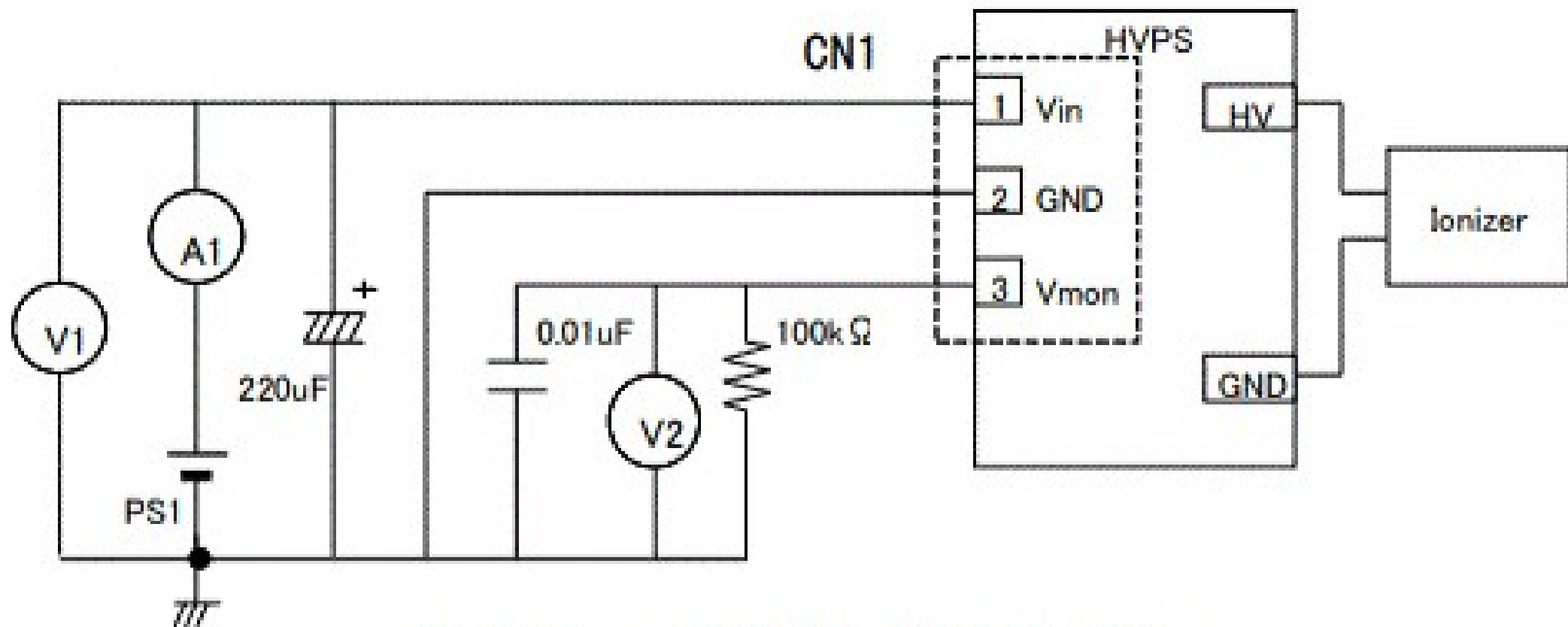
《 図 4 》 モニタ電圧試験回路(推奨回路)
