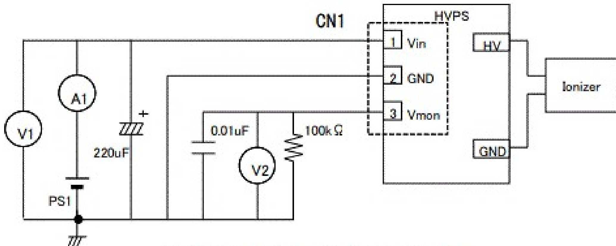
《 図 4 》 モニタ電圧試験回路(推奨回路)
