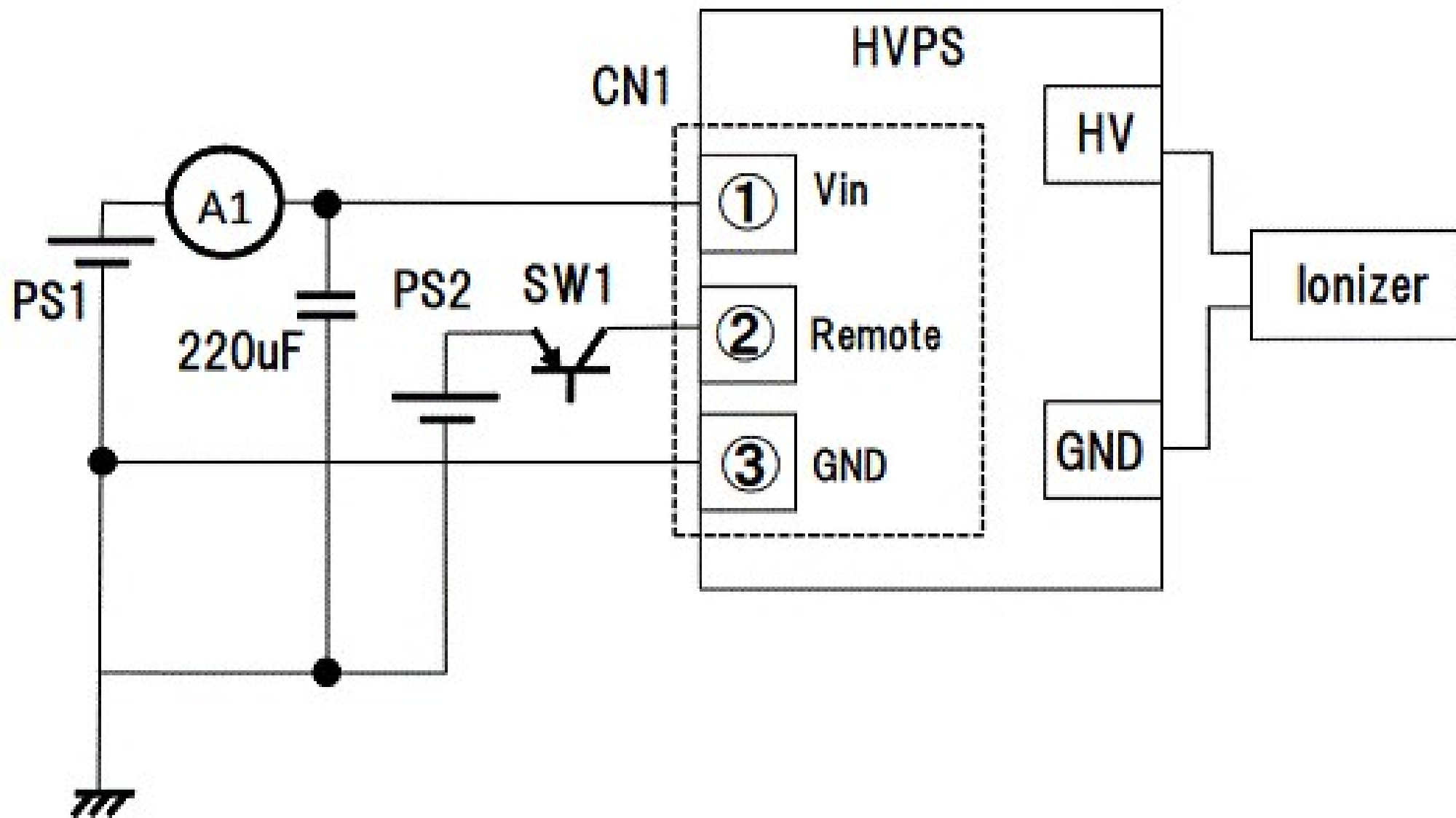
《 図 4 》 試験回路(推奨回路)
