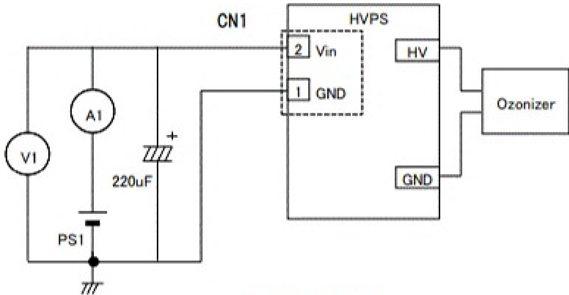
《 图 2 》 推奨回路
