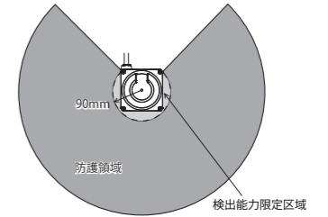
図-14. 検出能力限定区域
