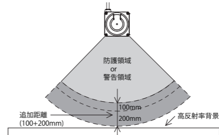
図-13. 高反射率背景でSE2Lを動作させるための追加距離
