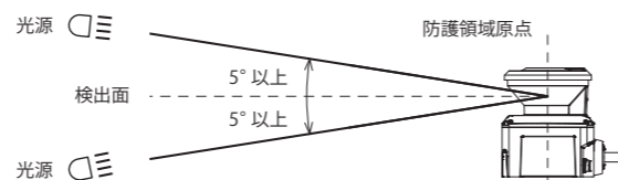
図-6. 外乱光対策の設置方法
