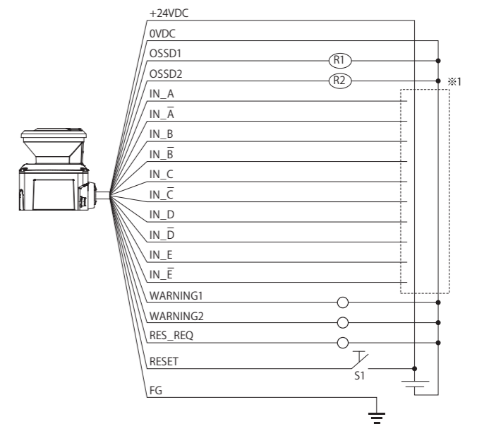
図-15. 配線例
