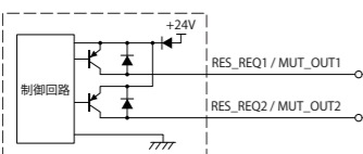
図-17. その他の出力回路
