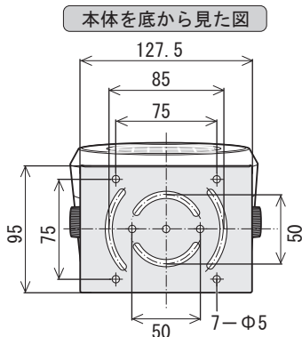
取付穴寸法図 (単位：mm)
