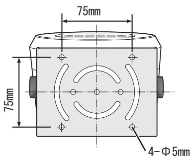
本体を底から見た図
