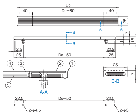
取付穴寸法詳細
