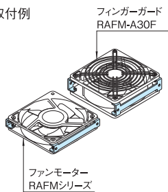
取付例
