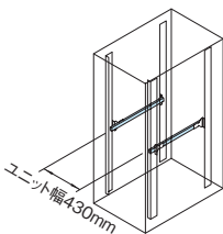
標準取付位置 ラック内部(ガイドレールブラケット)
