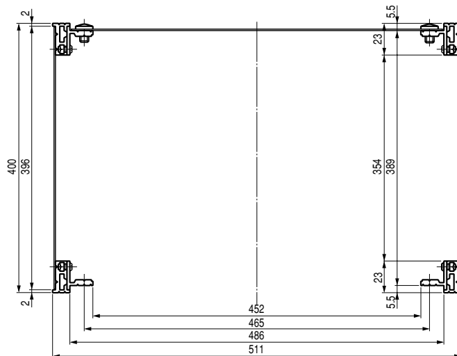
A-A矢視
