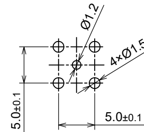
取り付け穴参考寸法
