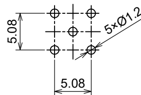
推奨 取付穴寸法
