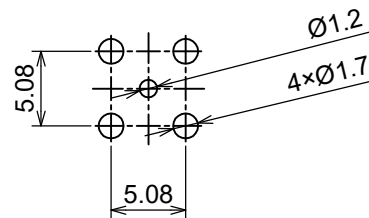
推奨 取付穴寸法
