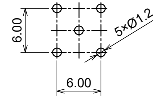
推奨 取付穴寸法
