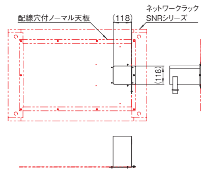
取付例
