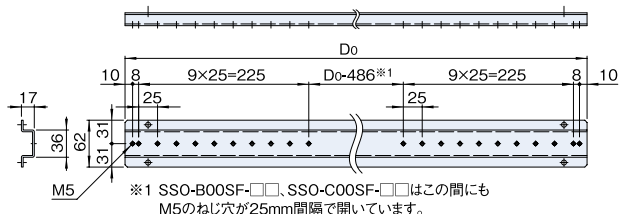
標準取付位置 ラック内
