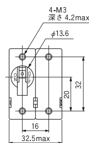
2極単ハンドル
