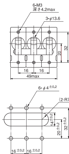
3極Hハンドル
