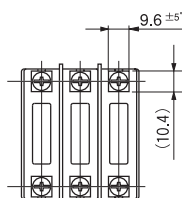
裏面図 (例)
