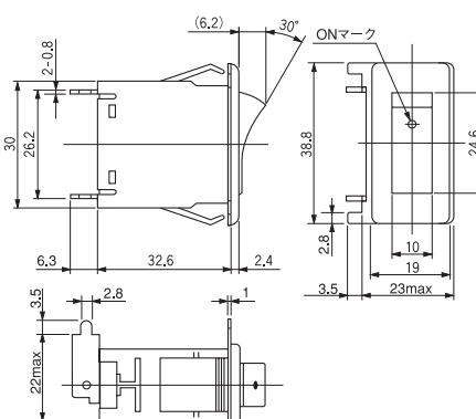
Bタイプ
