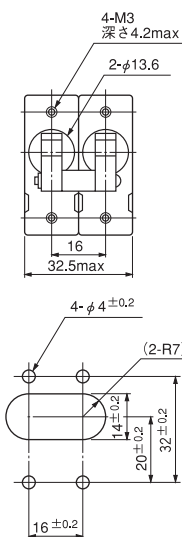
2極Hハンドル
