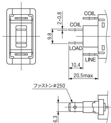
リレー型
