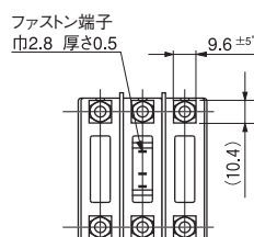
裏面図 (例)
