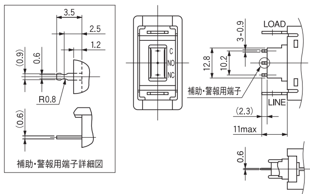
リレー型
