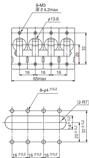
4極Hハンドル
