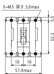
3極単ハンドル
