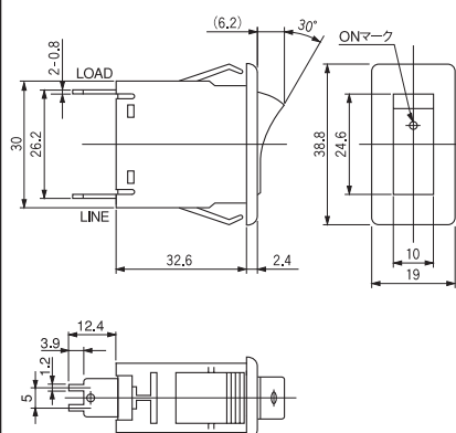
Dタイプ
