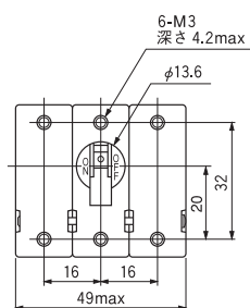
3極単ハンドル
