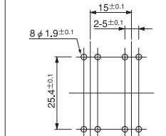
P板取付穴参考寸法
