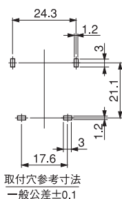
P板取付穴参考寸法図
