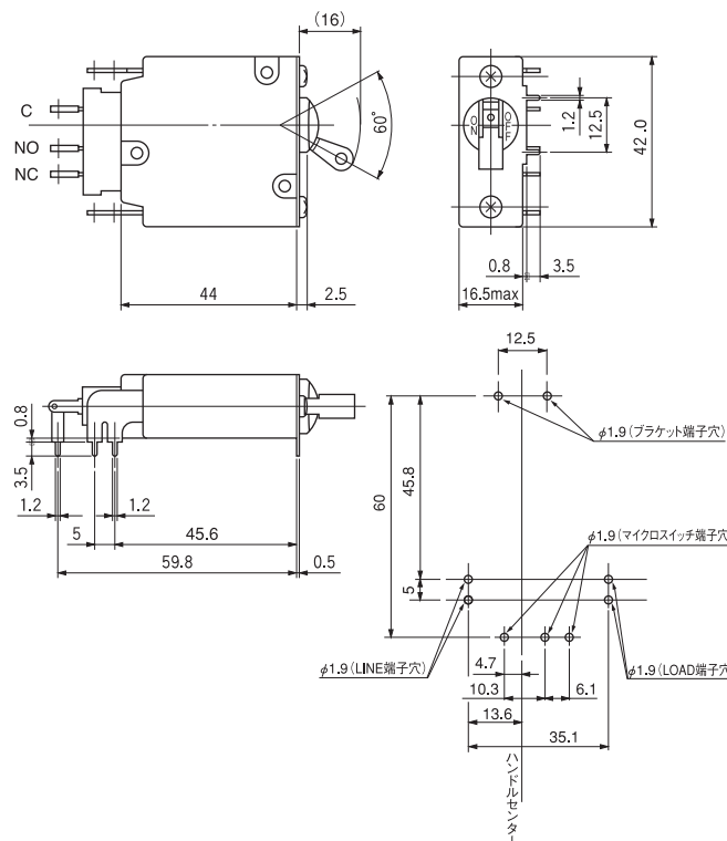
Aタイプ
