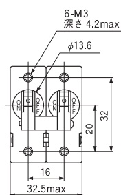
2極Hハンドル
