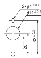
取付け穴寸法図
