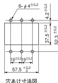
穴あけ寸法図
