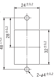
取付け穴寸法図
