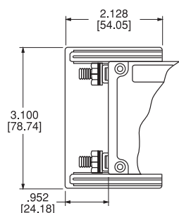
LELターミナルバリア (B)
