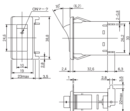
Aタイプ
