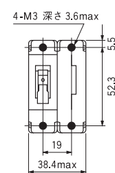
2極単ハンドル
