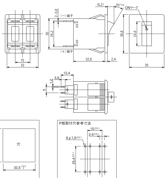
<SARPV-P-00-D>
