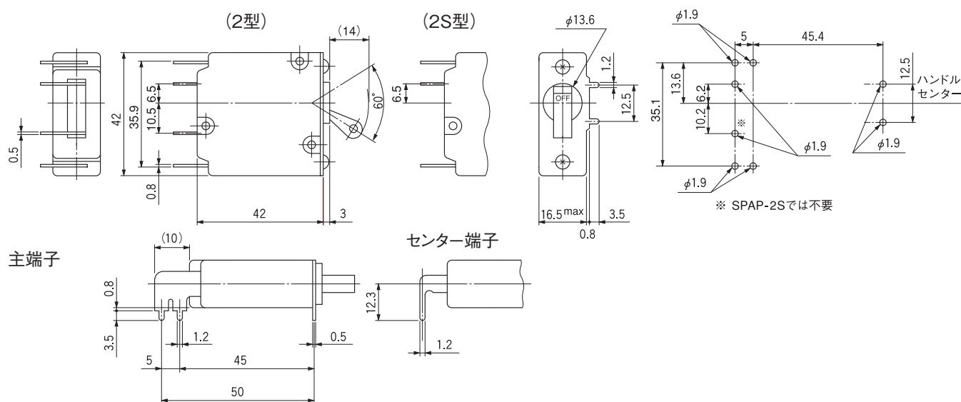
基板取付け穴寸法図
