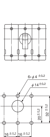
3極単ハンドル
