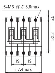
3極Hハンドル
