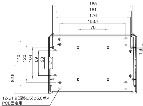
上下カバー内部 (VAA-14□□□□-WM1)
