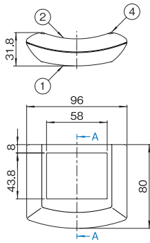
VGA-093-WM
