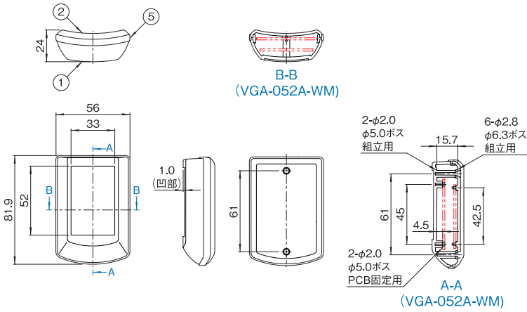
VGA-052A-WM
