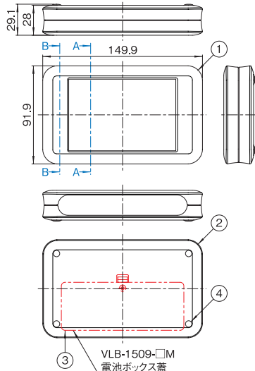
B-B (VLA-1509-□M)
