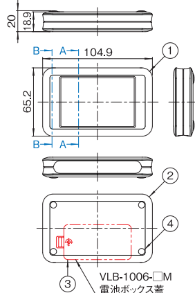
B-B (VLA-1006-□M)
