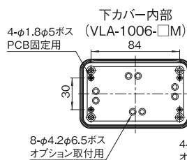
A-A (VLA-1006-□M)
