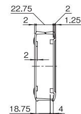
A-A (VLA-1509-□M)
