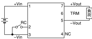
接続図
