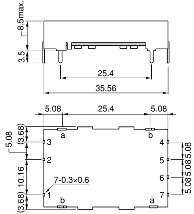
形状・寸法
