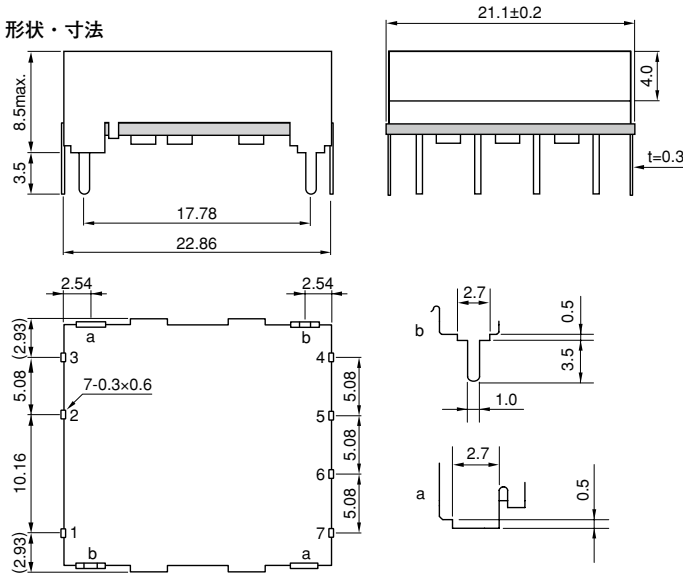
形状・寸法
