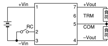
端子接続
