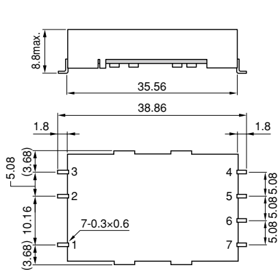
形状・寸法
