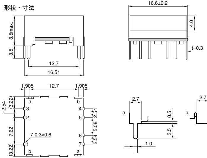
形状・寸法
