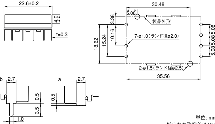
推奨基板取付け寸法
