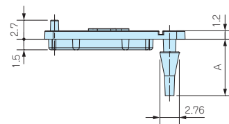
取付穴寸法図
