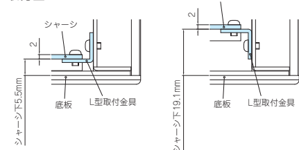
取付図
