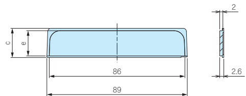
パネル寸法
