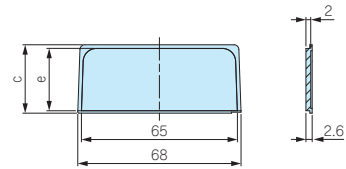
パネル寸法
