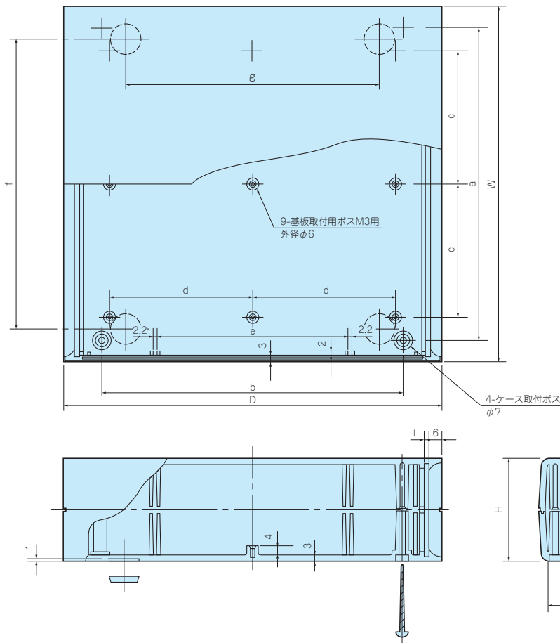
SY-190上面図
