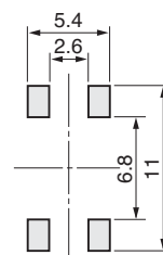
実装パターン寸法図 (スイッチ搭載側から見た図)
