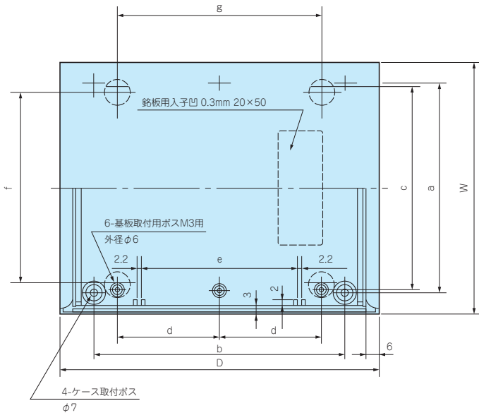
YX-110・150上面図
